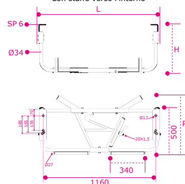
With inwards brackets Con staffe verso l'interno
