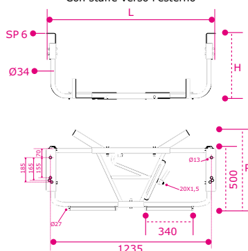
With outwards brackets Con staffe verso l'esterno
